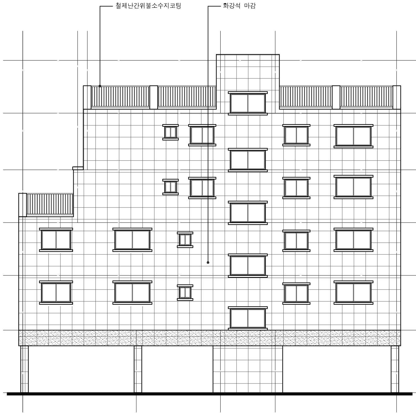
배 면 도 SCALE : A3 : 1/120
