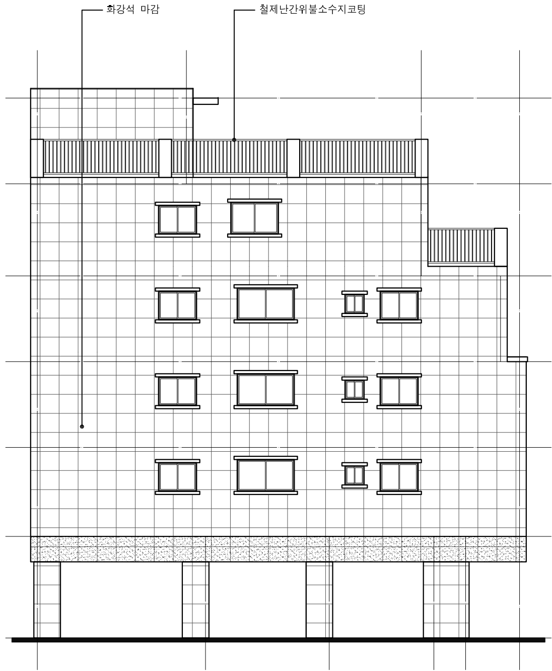
좌 측 면 도 SCALE : A3 : 1/120
